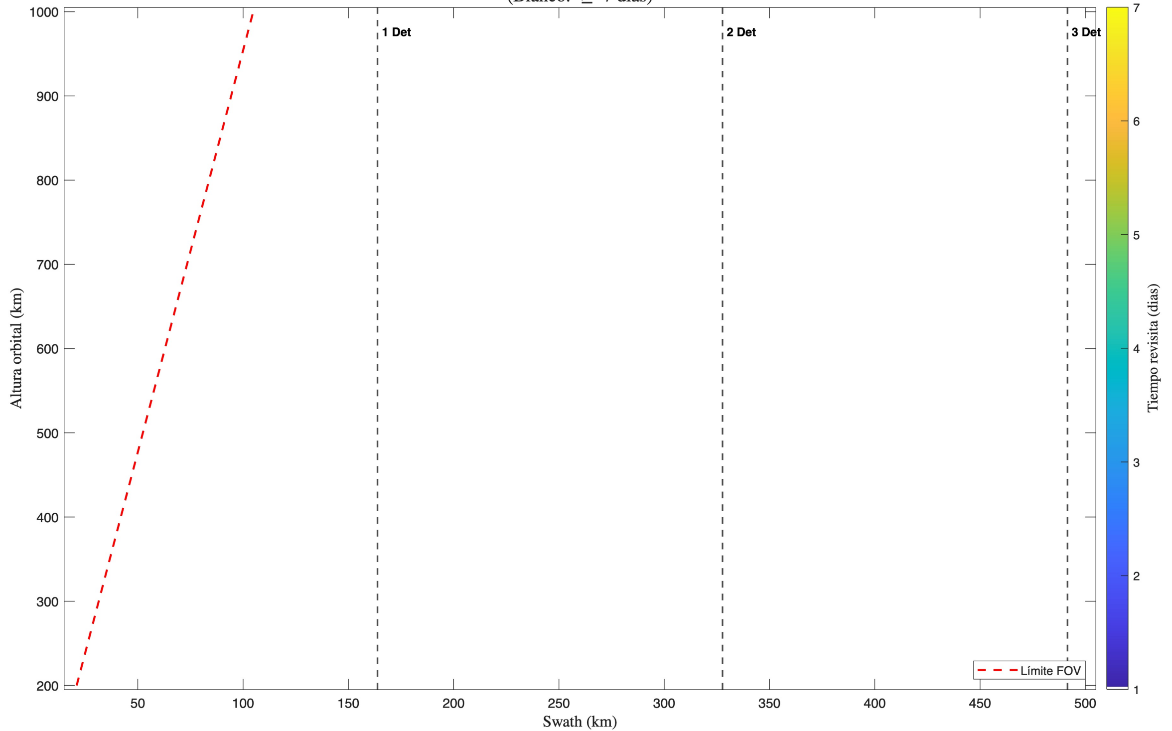
Tiempo Revisita - 2 Satelite(s); 2 Telescopio(s): Cassegrain; Detector 2 (Blanco: \geq 7 dias)
